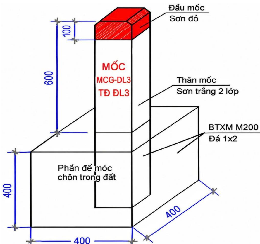
Hình 2. Quy cách mốc chỉ giới bảo vệ đập theo thông tư 08/2026/TT-BNNMT
